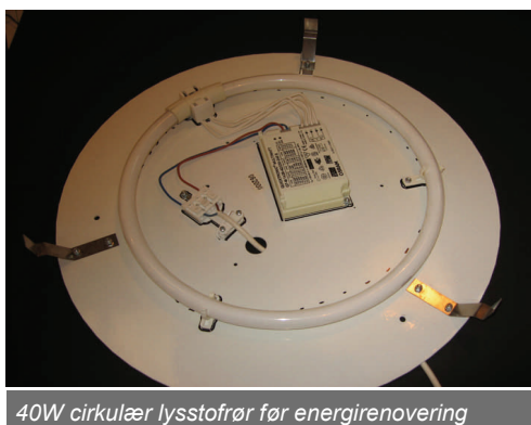
40W cirkulær lysstofrør før energirenovering
