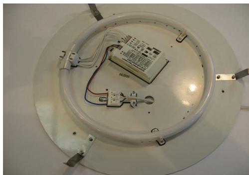
Indbygget cirkulær lysstofrør før energioptimering
